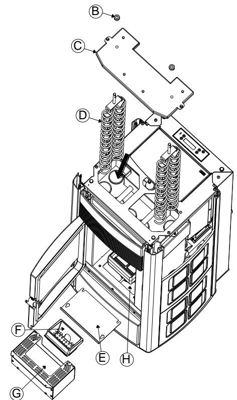
Figura 16 – Limpieza del haz de tubos, turbuladores y compartimento inferior (EGO-STAR)
