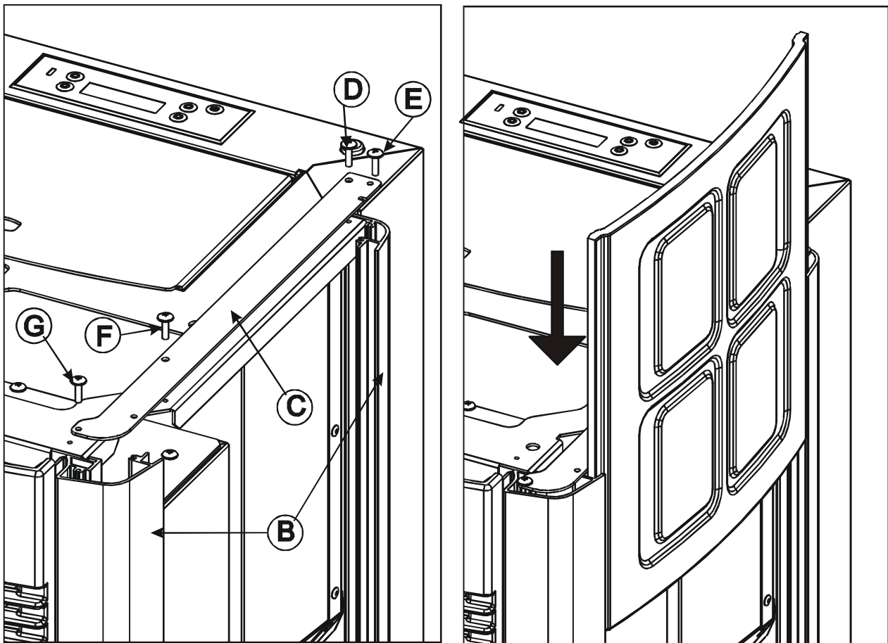
Figura 7 - Costados estufa STAR
