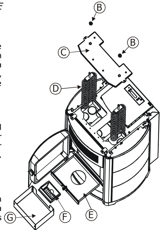
Figura 16a – Limpieza del haz de tubos, turbuladores y compartimento inferior (SUITE/CLUB/MUSA)
