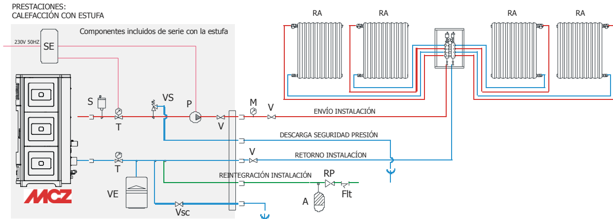
CONFIGURACIÓN: STAR/EGO/SUITE/CLUB/MUSA SIN KIT SANITARIO ESQUEMA INSTALACIÓN CON DEPÓSITO CERRADO SOLO DE CALEFACCIÓN MEDIANTE RADIADORES
