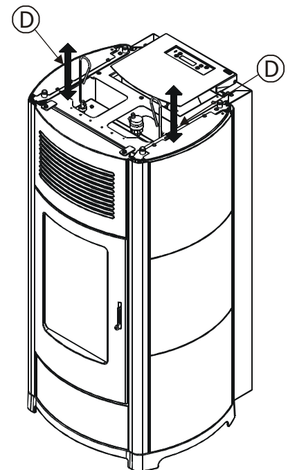
Figura 15A – Limpieza del haz de tubos interno mediante rasquetas (SUITE-CLUB-MUSA)
